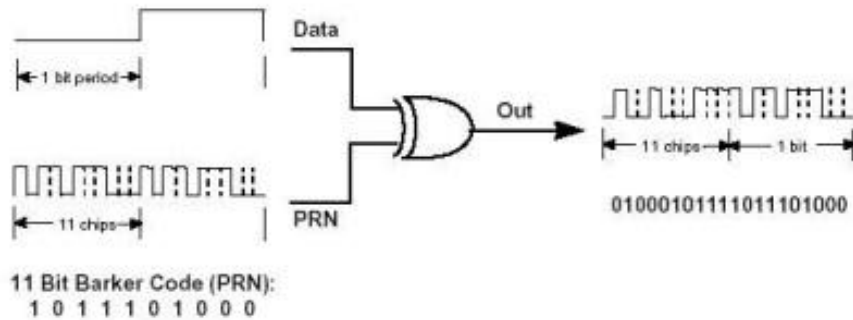
شکل ۲.۱۲: مدار مدولاسیون با استفاده از کدهای بارکر
