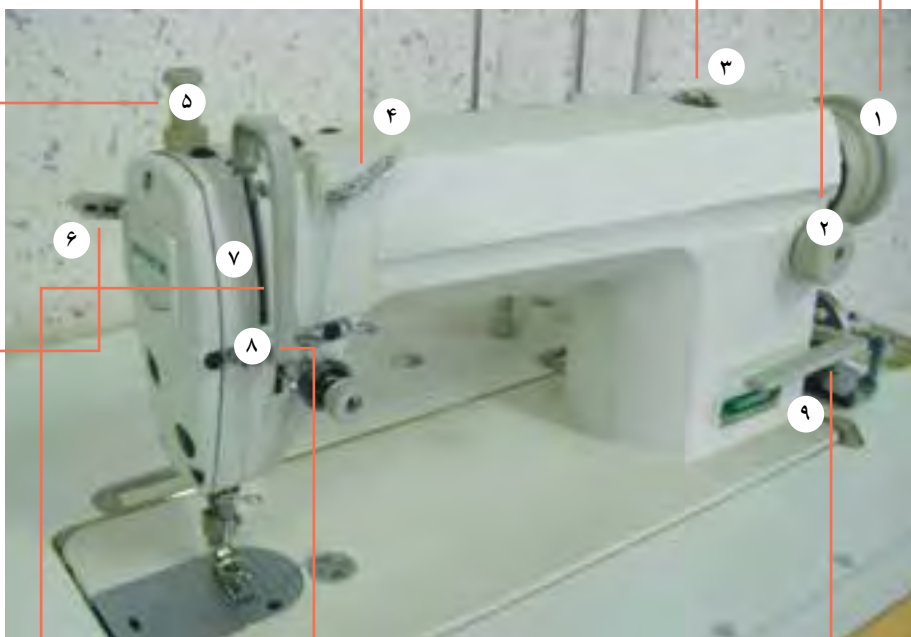
۴- گیره نخ
