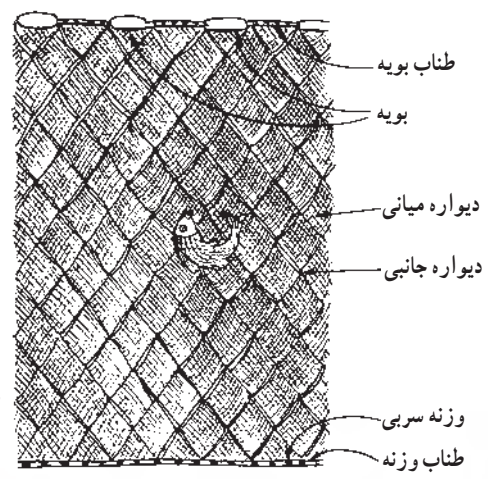
شکل ۳-۳- تور سه لایه یا تور ترامل
