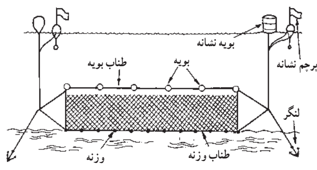
شکل ۲-۳- تور گوشگیر عمقی ثابت
