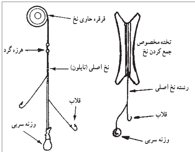
شکل ۱-۴- نمونه قلاب دستی ساده
