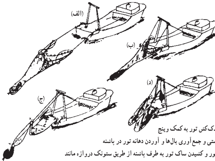
شکل ۱۱-۱- مراحل مختلف جمع‌آوری تور ترال در یک شناور تراولر باشنه کش
