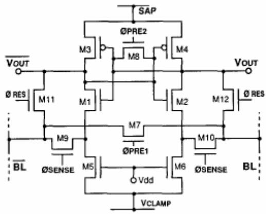
شکل 31 : sense amplifier در مرجع [19]
