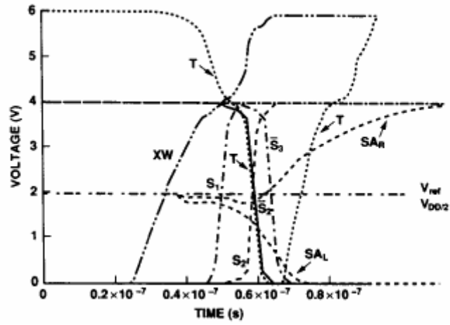
شکل 34 : شکل موج ولتاژ نقاط مختلف در مدار شکل 33
