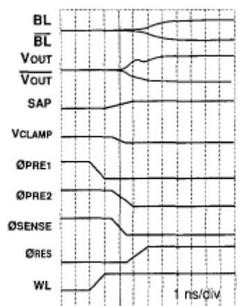
شکل 32 : شکل موج ولتاژ نقاط مختلف در مدار شکل 31
