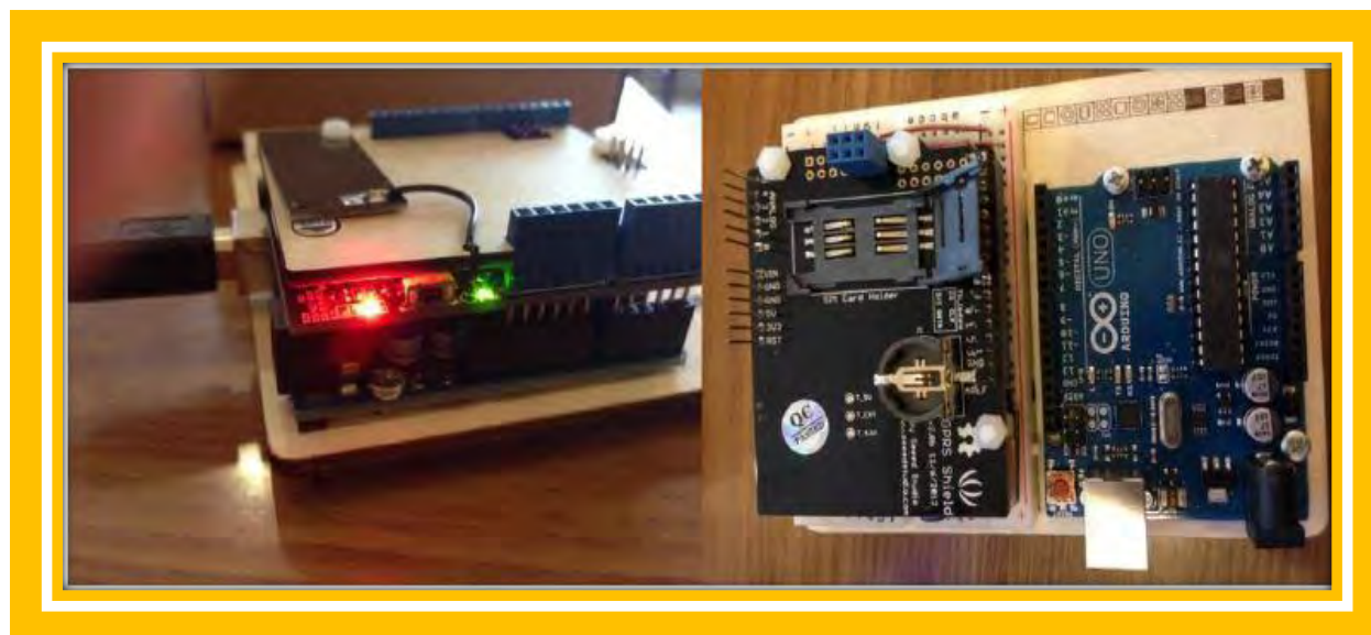
تصویر 30 میکروکنترلر Arduino و مودم GSM برنامه پذیر SIM900
