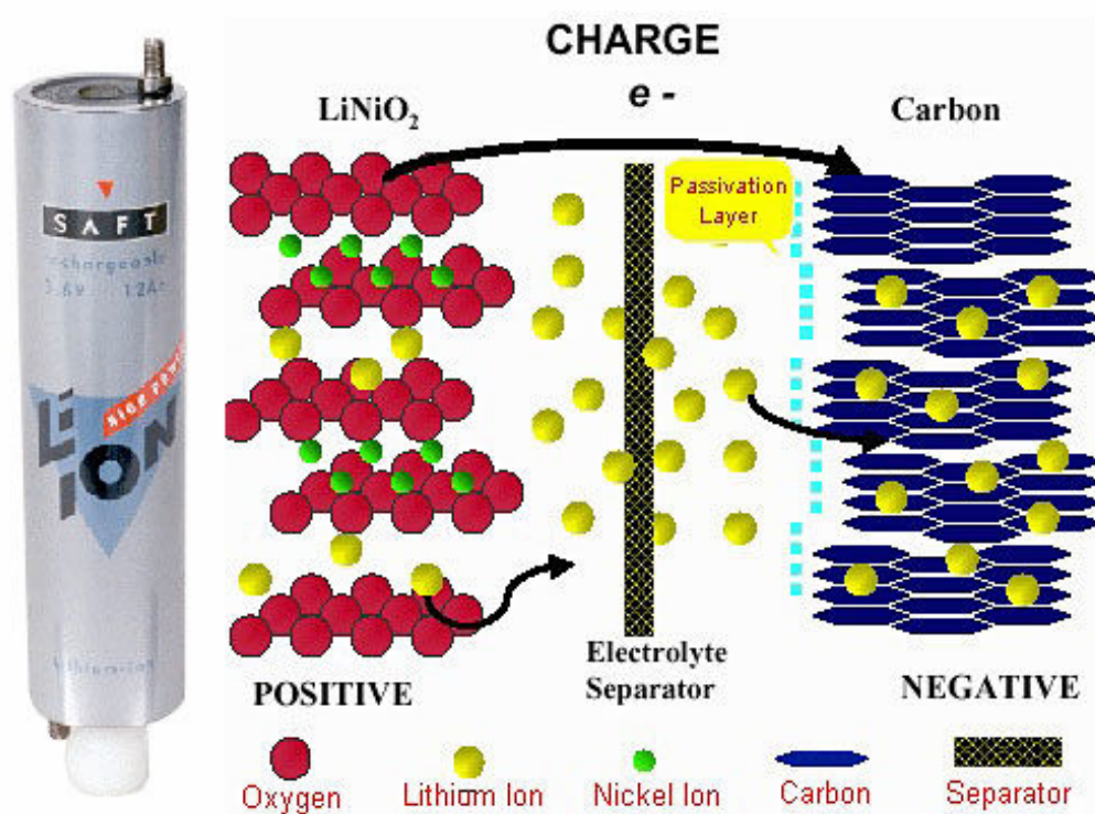
شکل ۲-۲- ساختار باتری Li-ON
