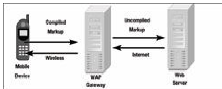
شکل ۹-۲ - WAP Gateway
