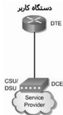
استفاده از اینترفیس WAN (منبع: سایت سیسکو)
